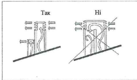
Рисунок 5. Закінчення димоходу
