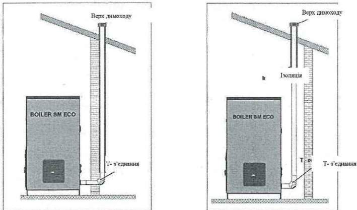
Рисунок 3а і 3б. Викиди димових газів
