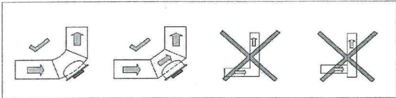
Рисунок 4 б. Рекомендовані коліна витяжних труб
