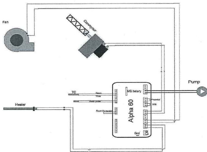
Рисунок 30. СХЕМА ЕЛЕКТРОСИСТЕМИ
