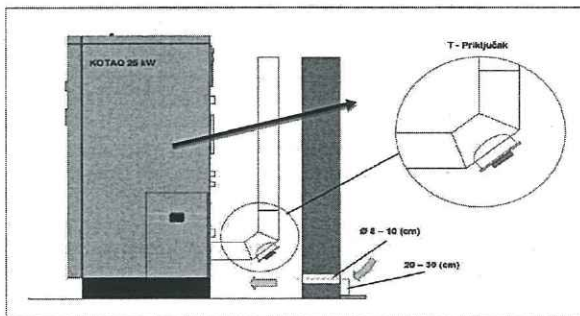
Рисунок 10. Мінімальні отвори для встановлення вентиляційних решіток
